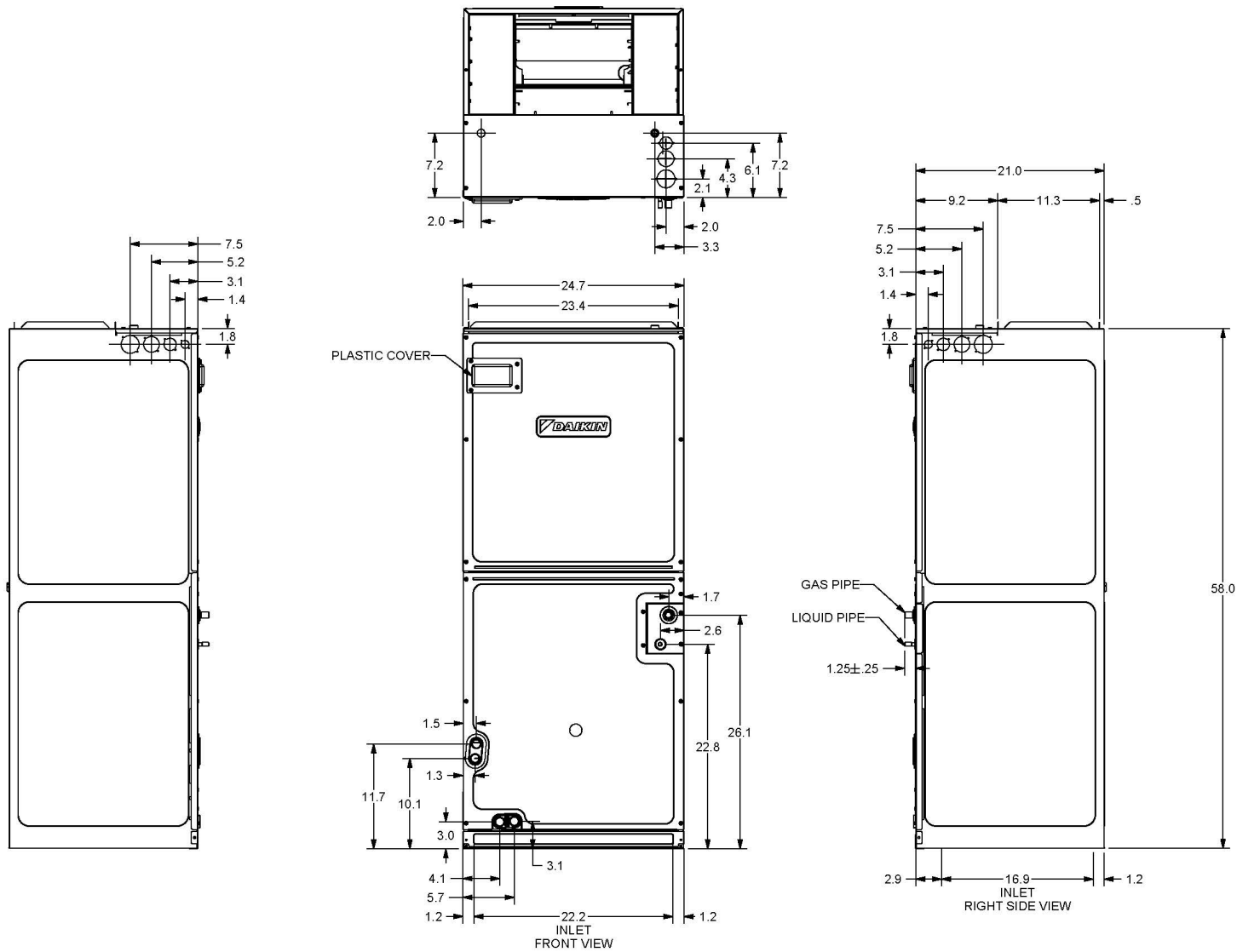
FXTQ54/60 TAVJU
